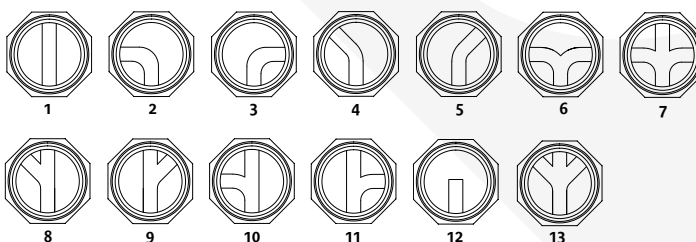
• Regard DN 1000 avec cunette incorporé pour 200 PVC CR8 - hauteur utile : 0,48
